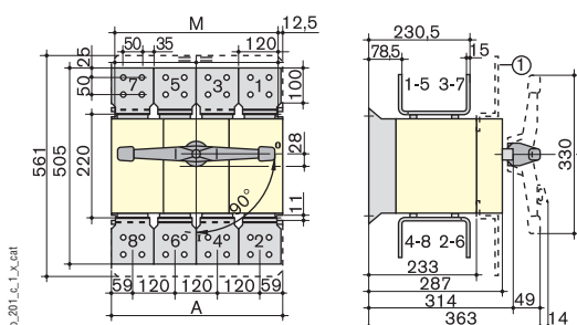
1. Клеммные крышки.
