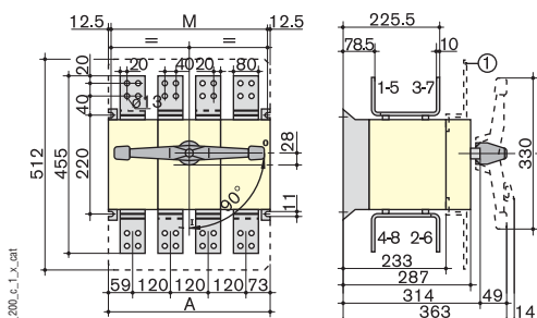
1. Клеммные крышки.
