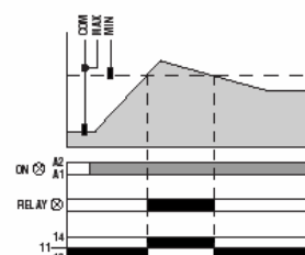
2-х электродная схема
