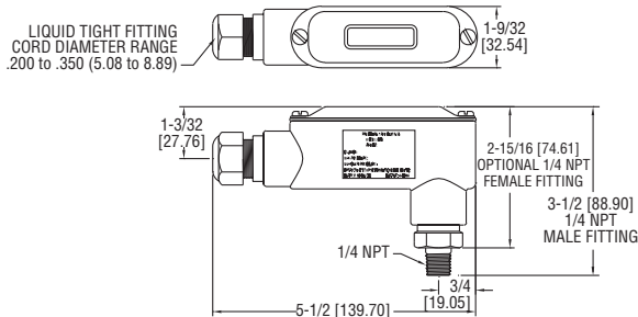
-CH Conduit Housing
