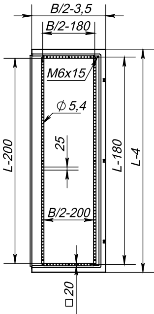
Дверь левая, вид изнутри
