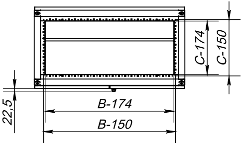
Вид сверху (без верхней панели)
