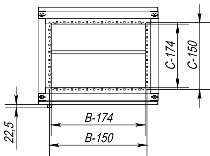
Вид сверху (без верхней панели)
