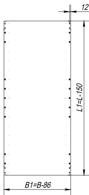
Панель монтажная
