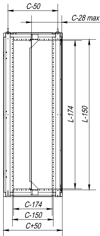
Вид слева, разрез
