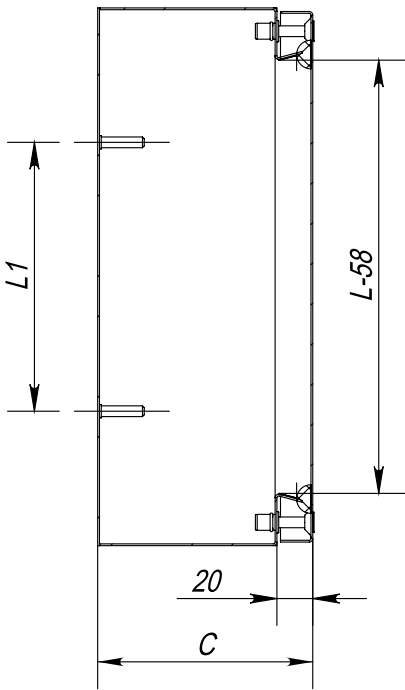
Вид слева, разрез
